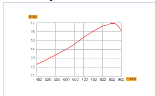
Radiationsdiagramm
