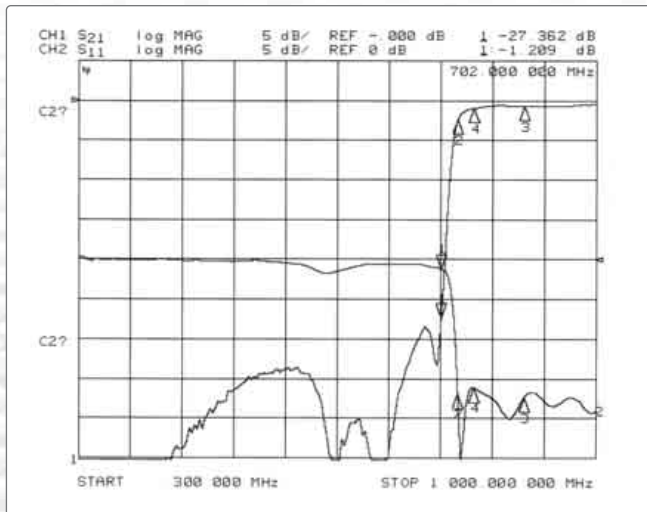
BK 702/734: Durchgangs- und Rückflussdämpfung 734-862 MHz BK 702/734: through loss and return loss 734-862 MHz
